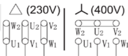
Fig. 6: Переключение Y-Δ
